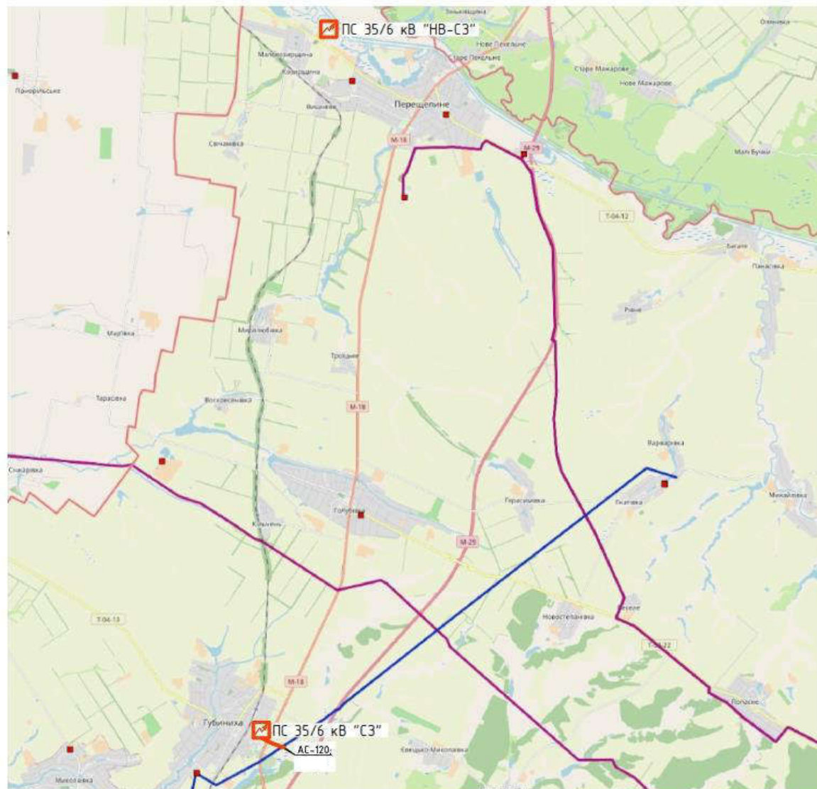
Рис. 13. Карта-схема електричних мереж 35-150 кВ в районі розміщення ПС 35/6 "СЗ", ПС 35/6 "НВ-СЗ" 2021 рік
