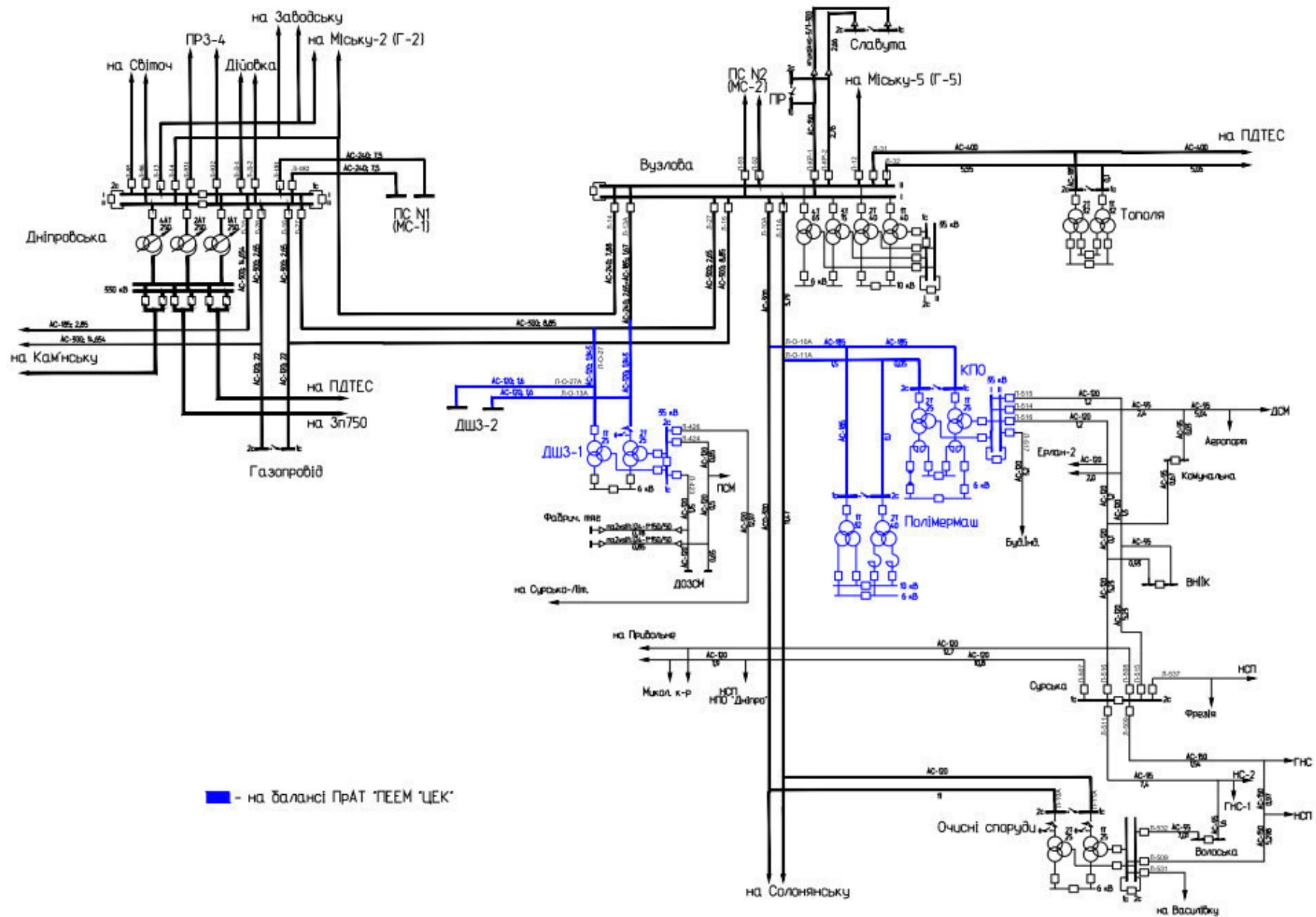
Рис.1. Схема електричних з'єднань мереж 35-150 кВ в районі розміщення ПС 150/35/6 кВ "КПО", ПС 150/10/6 кВ "ПІЛМ" та ПС 150/35/6 кВ "ДШЗ-1" 2021 рік
