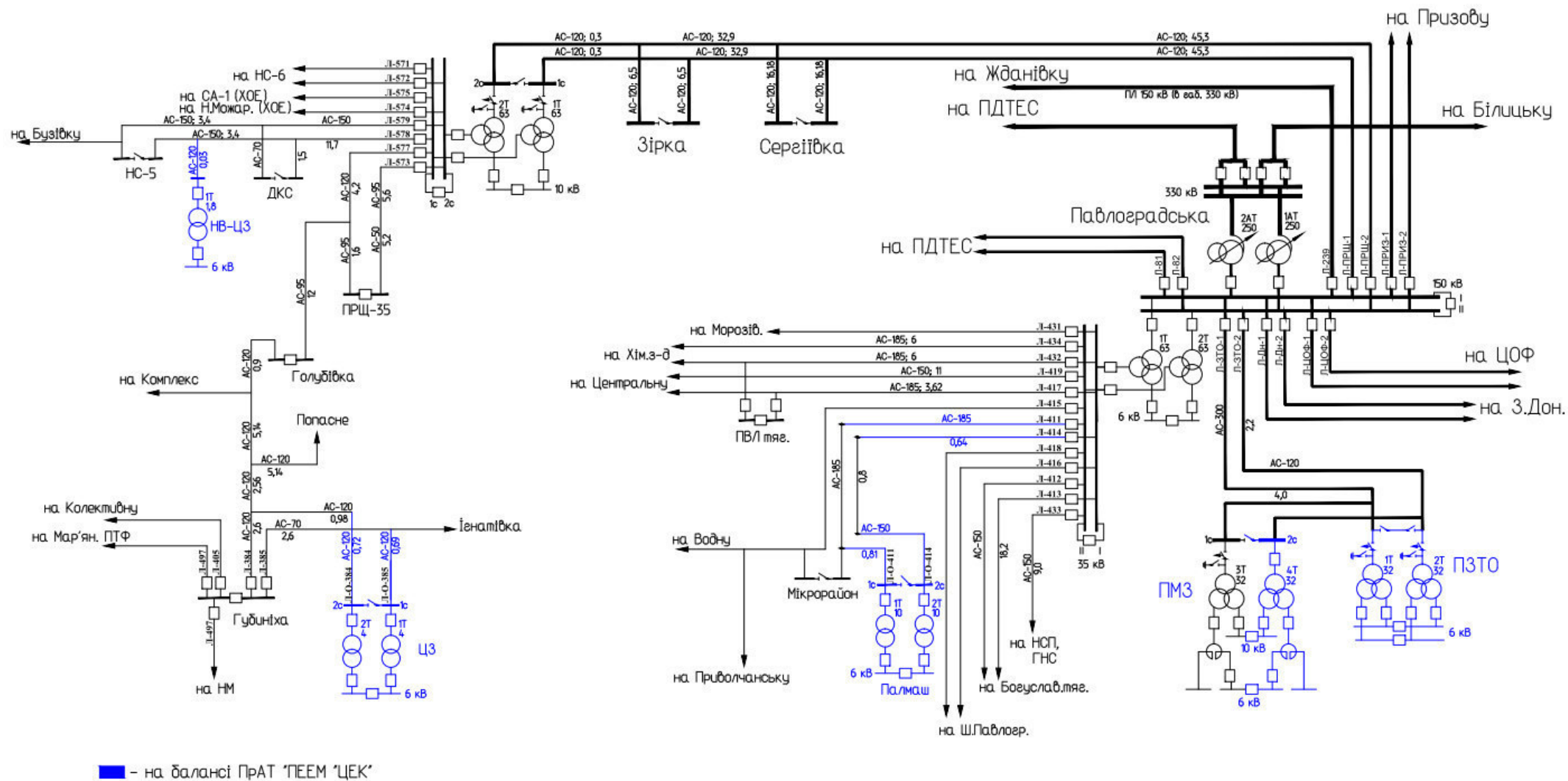
Рис.8. Схема електричних з'єднань мереж 35-150 кВ в районі розміщення ПС 150/6/10 кВ "ПМЗ" та ПС 150/6/6 кВ "ПЗТО", а також ПС 35/6 кВ "Палмаш", ПС 35/6 кВ "ЦЗ" та ПС 35/6 кВ "НВ-ЦЗ" 2026 рік
