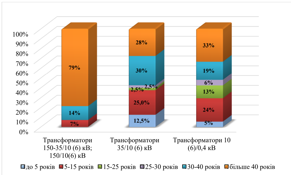
Рис. 16.1. Технічний стан силових трансформаторів
