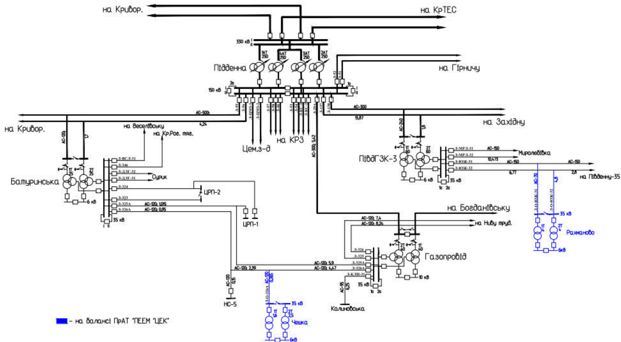
Рис.15.Схема електричних з'єднань мереж 35-150 кВ в районі розміщення ПС 35/6 кВ "Ражманово" та ПС 35/6 кВ "Чешка" 2021 рік
