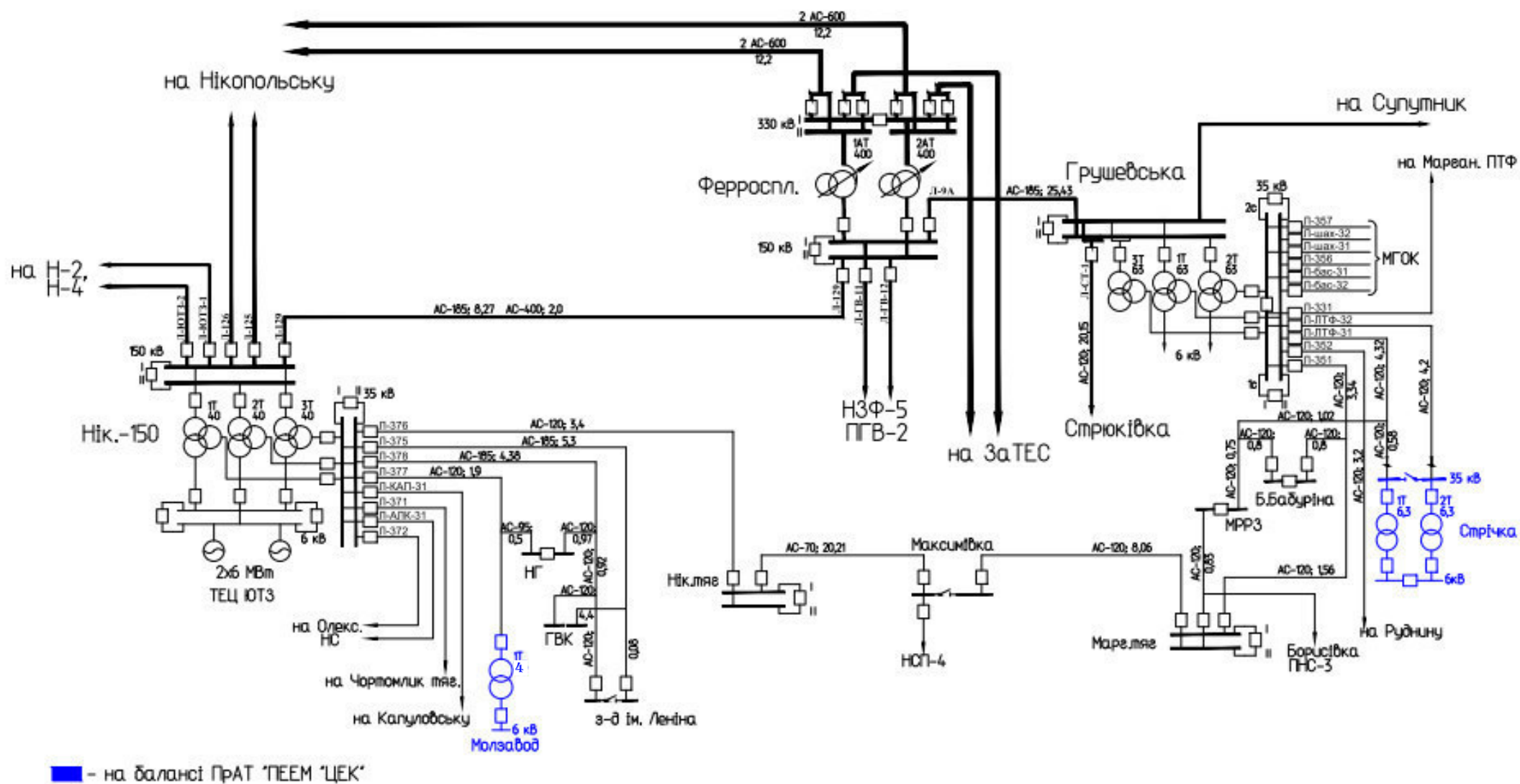
Рис.20. Схема електричних з'єднань мереж 35-150 кВ в районі розміщення ПС 35/6 кВ "Стрічка" та ПС 35/6 кВ "Молзавод"
