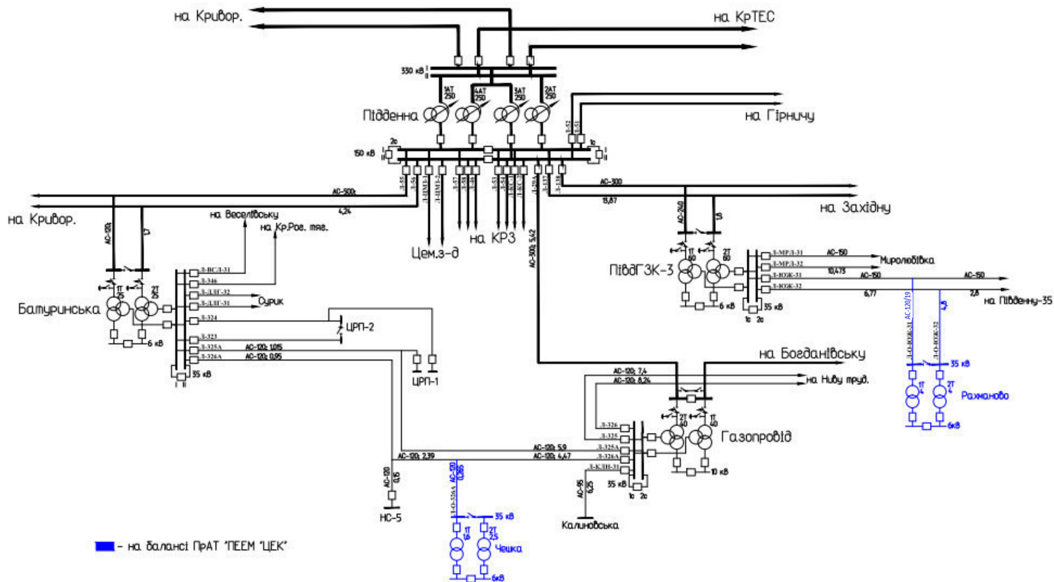
Рис.16.Схема електричних з'єднань мереж 35-150 кВ в районі розміщення ПС 35/6 кВ "Ракманово" та ПС 35/6 кВ "Чешка" 2026 рік
