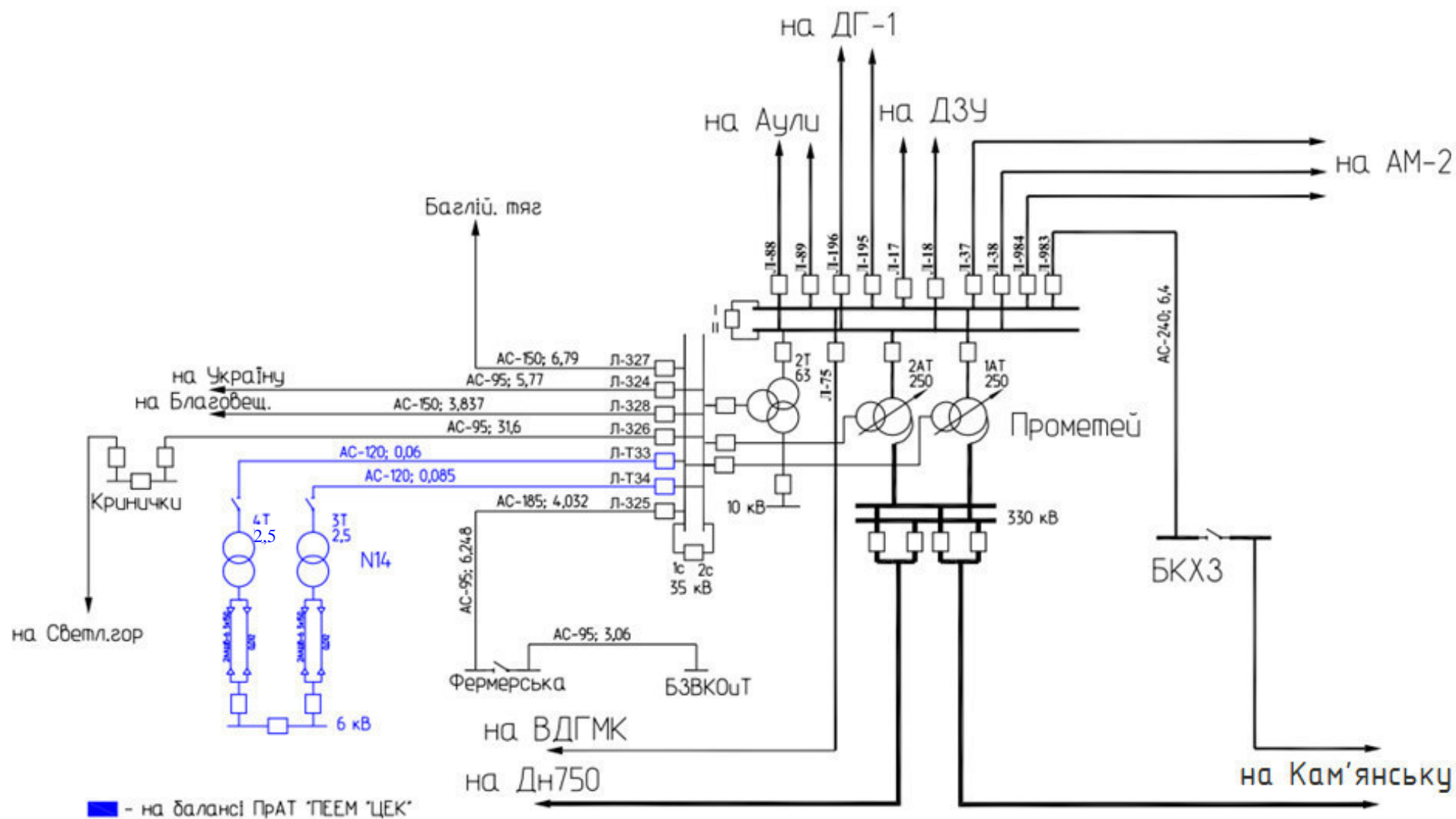
Рис. 21. Схема електричних з'єднань мереж 35-150 кВ в районі розміщення ПС 35/6 кВ N14 2021 рік
