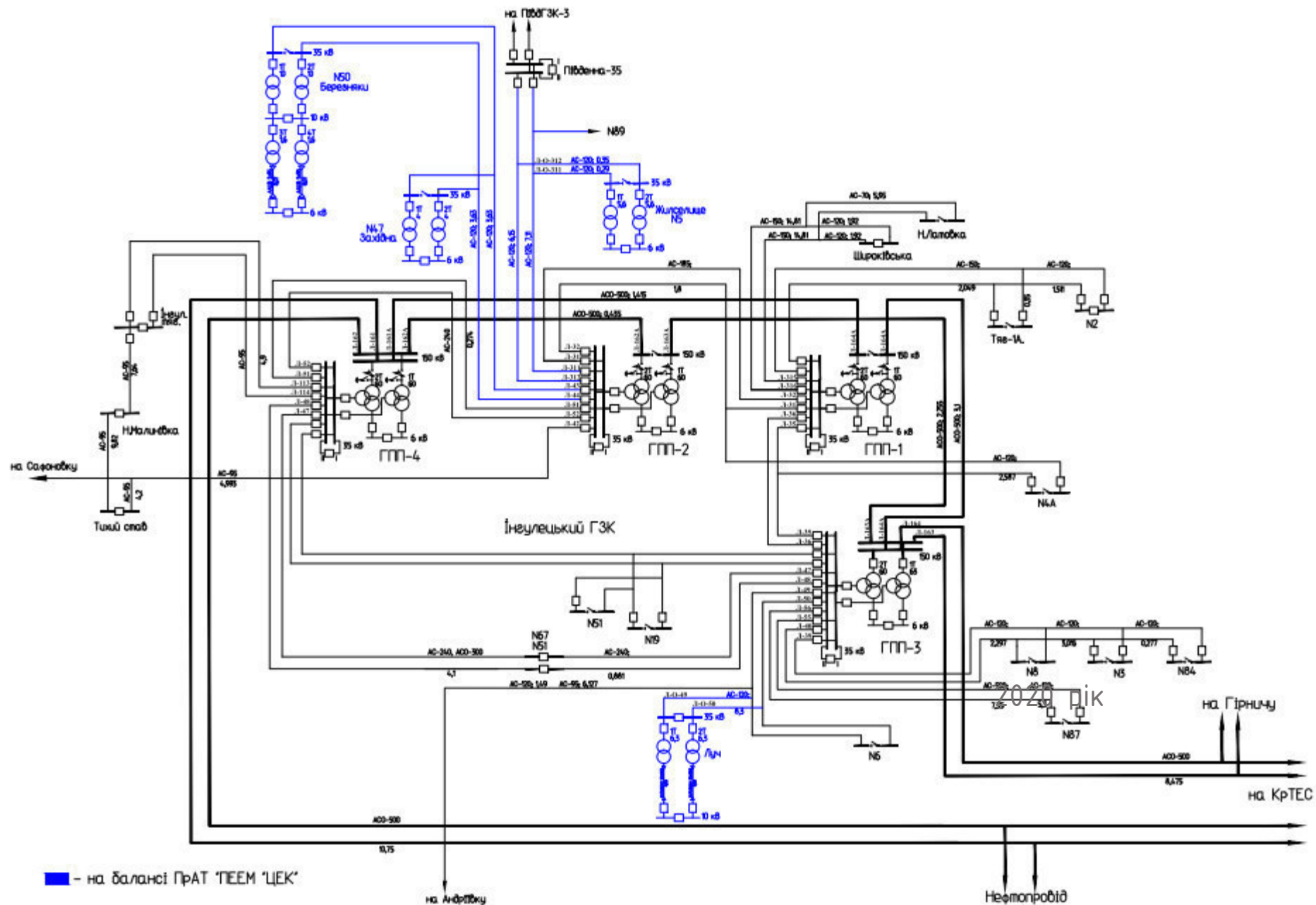
Рис.13.Схема електричних з'єднань мереж 35-150 кВ в районі розміщення ПС 35/6 кВ N5 "Жилоселище", ПС 35/6 кВ N47 "Західна", ПС 35/10/6 кВ N50 "Березняки" та ПС 35/10 кВ "Лун" 2021 рік
