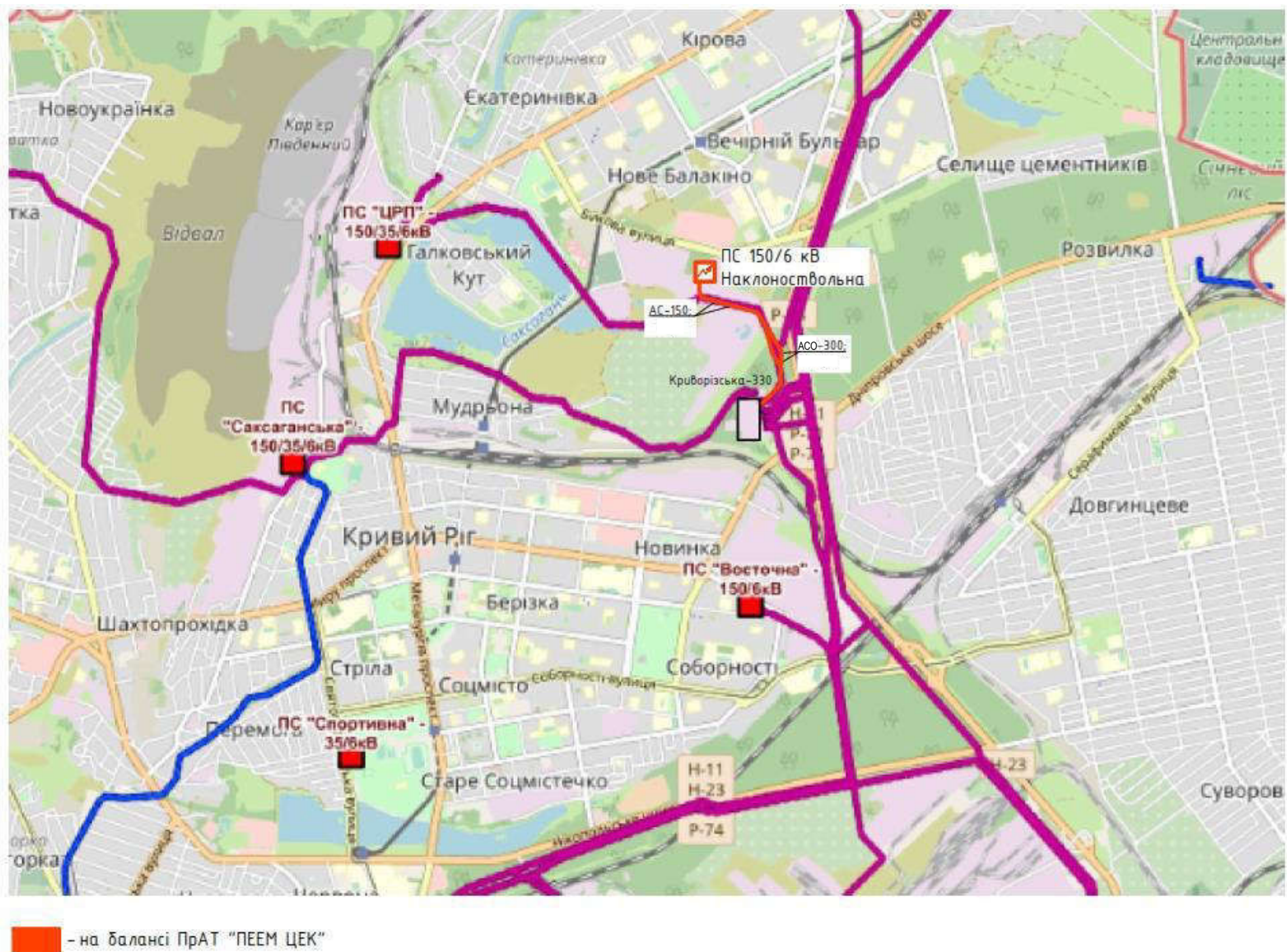
Рис. 15. Карта-схема електричних мереж 35-150 кВ в районі розміщення ПС 150/6 кВ "Наклоноствольна" 2021 рік
