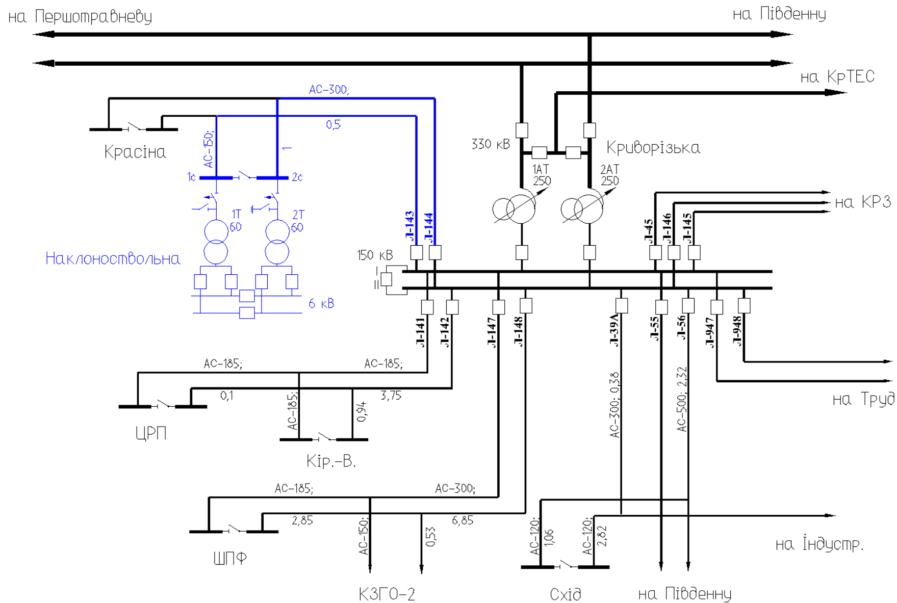
Рис.9.Схема електричних з'єднань мереж 35-150 кВ в районі розміщення ПС 150/6 кВ "Наклоноствольна"2021 рік
