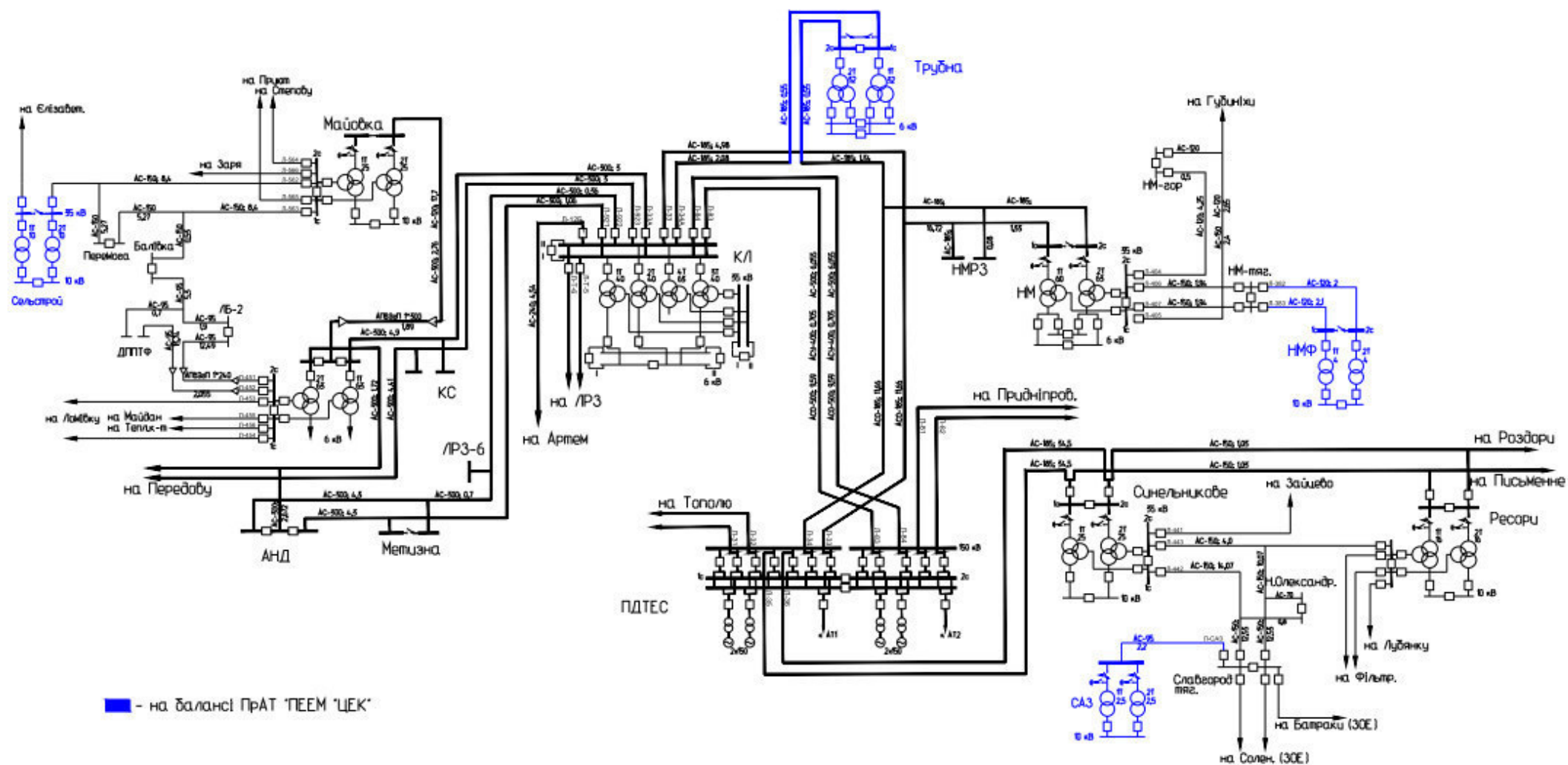
Рис.4. Схема електричних з'єднань мереж 35-150 кВ в районі розміщення ПС 150/6/6 кВ "Трубіна" та ПС 35/10 кВ "НМФ", ПС 35/10 кВ "САЗ", ПС 35/10 кВ "Сельстрой" 2026 рік
