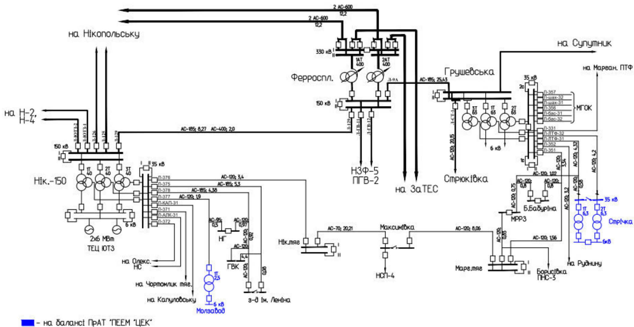
Рис.19. Схема електричних з'єднань мереж 35-150 кВ в районі розміщення ПС 35/6 кВ "Стрічка" та ПС 35/6 кВ "Молзавод"
