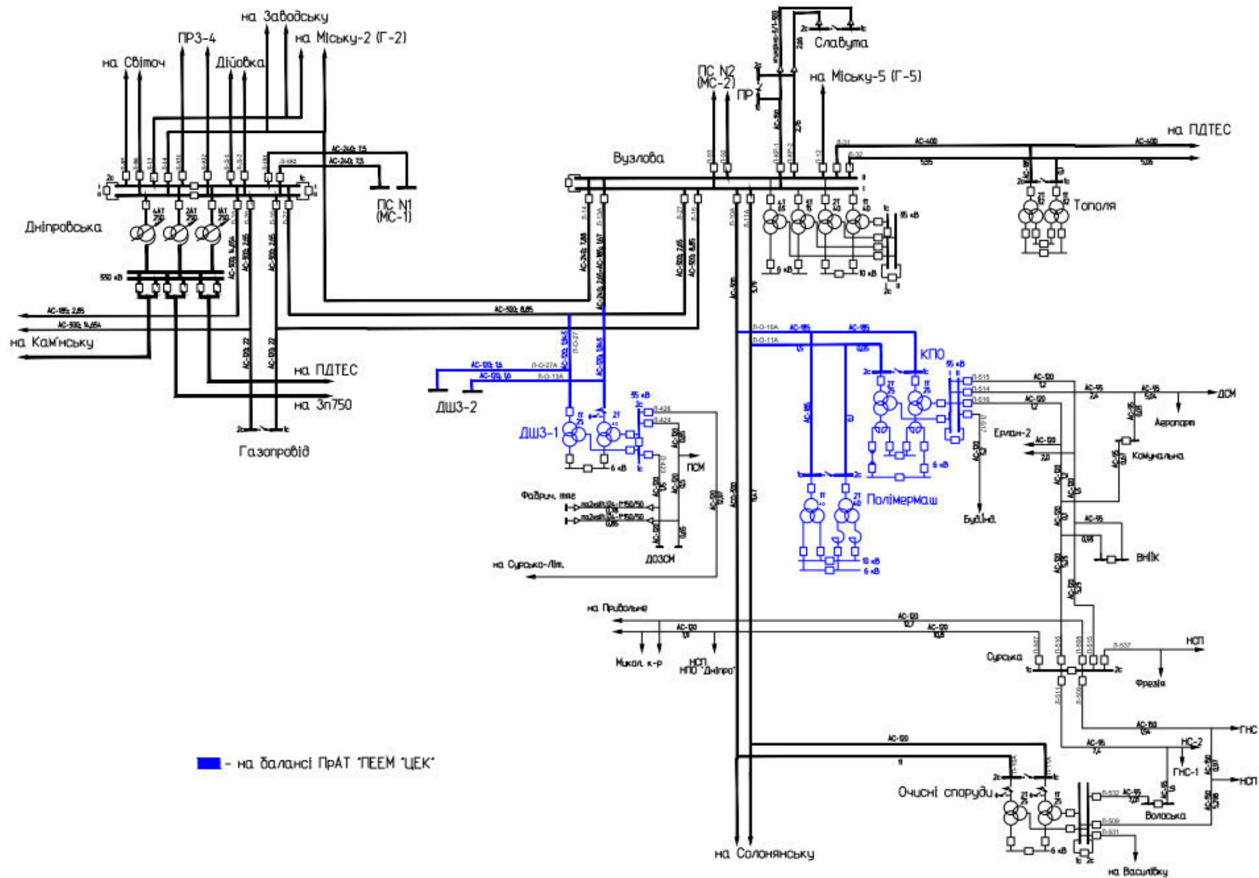
Рис.2. Схема електричних з'єднань мереж 35-150 кВ в районі розміщення ПС 150/35/6 кВ "КПО", ПС 150/10/6 кВ "ПІЛМ" та ПС 150/35/6 кВ "ДШЗ-1" 2026 рік
