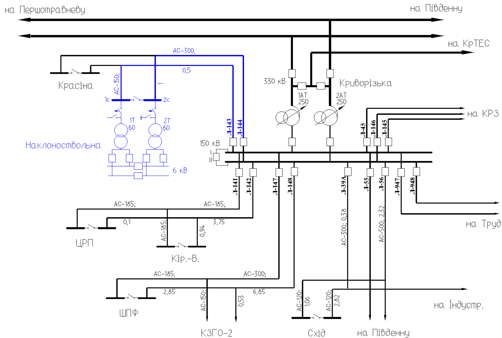
Рис.10. Схема електричних з'єднань мереж 35-150 кВ в районі розміщення ПС 150/6 кВ "Наклоноствольна" 2026 рік
