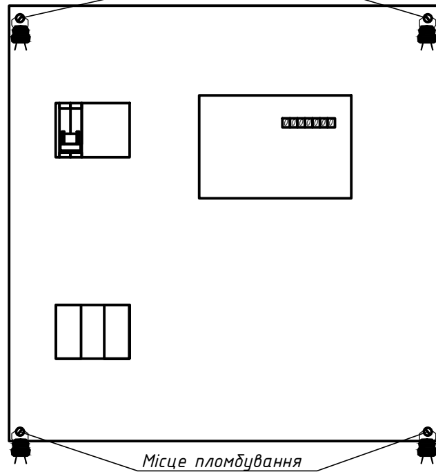
Шафа обліку ШО (зовнішні двері не показані) Місце пломбування
