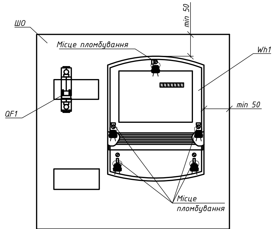
Шафа обліку ШО (зовнішні двері та захисна панель не показані)
